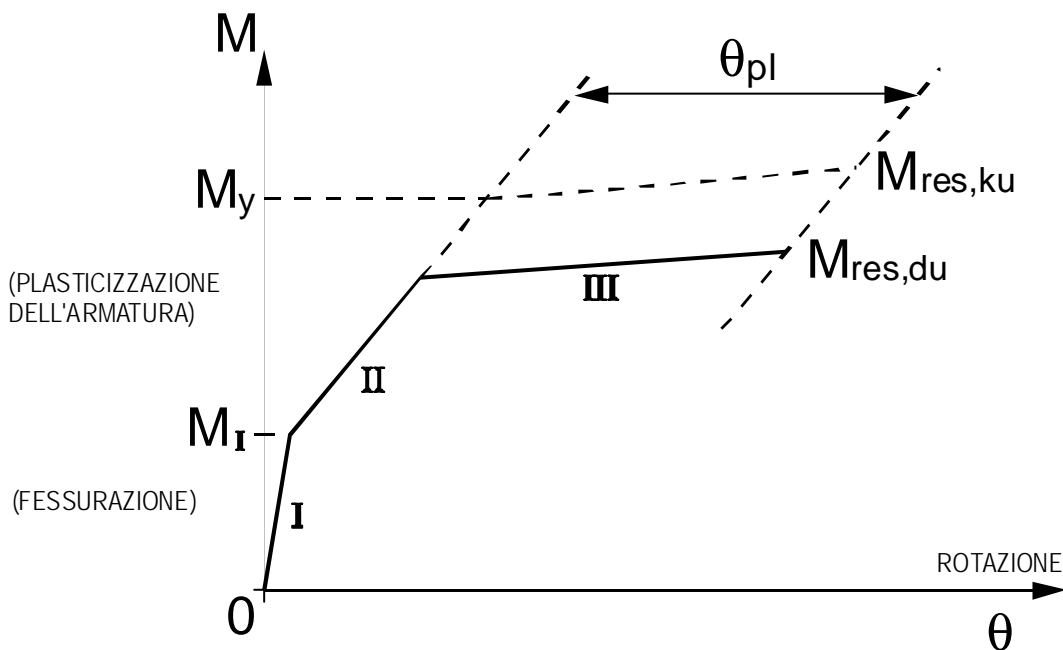
Fig. 1 - Diagramma momento-rotazione: idealizzazione tri-lineare
