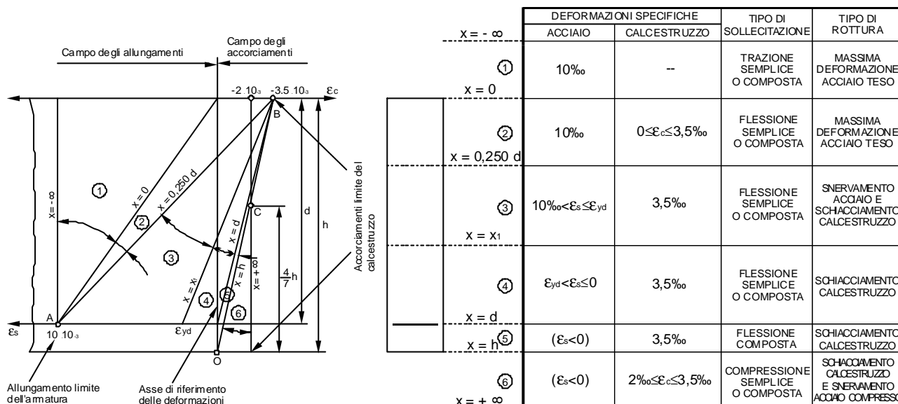
Fig. 2 - Diagramma di deformazione allo stato limite ultimo
