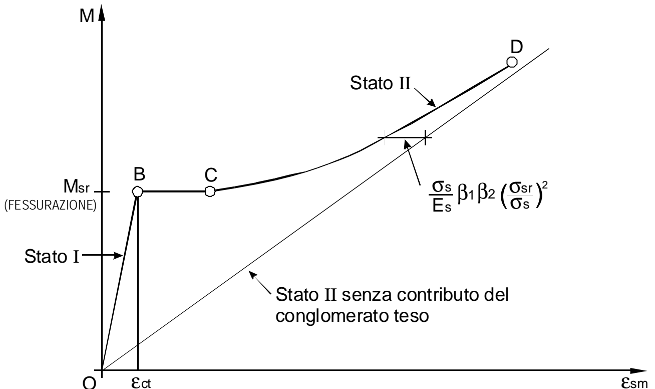
Fig. 6 - Diagramma M - \epsilon_{sm}
