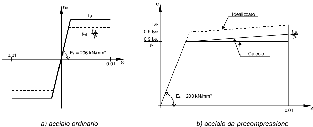
Fig. 3 - Diagramma di calcolo s - e
