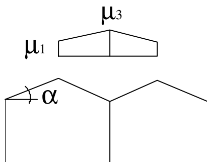
Fig. 6.5 - Condizione ulteriore di carico per coperture a pi• campate
